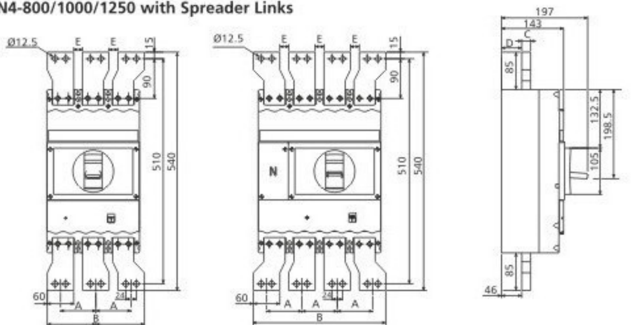
3P Frame
